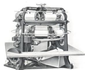
23. ábra. Maratti-gép [31]
